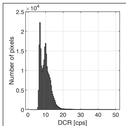
暗计数分布
