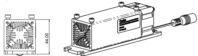
LaserBoxx optional heatsink
