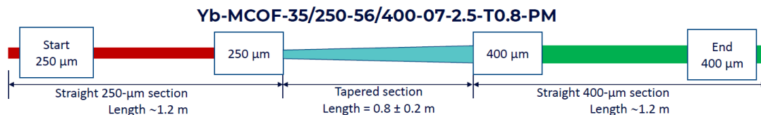
图 1、锥形掺镱光纤结构示意图
