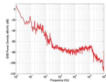
激光的相位噪声谱密度
